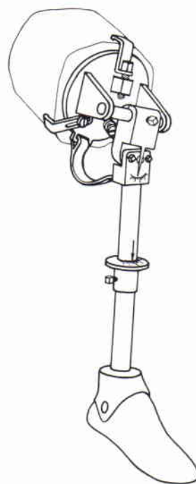
Fig. 7. Schneider's "Gehmaschine."
